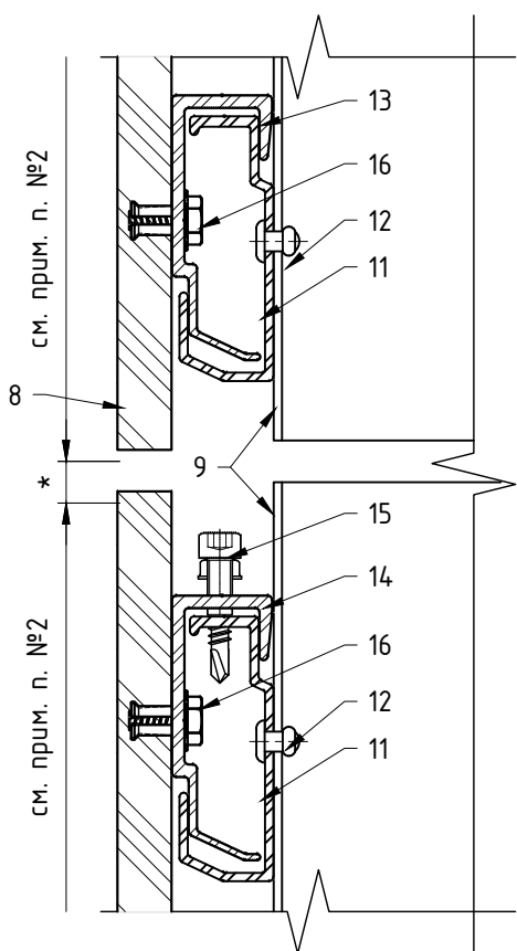
Фрагмент №1 (вариант с MFT-HP E)
