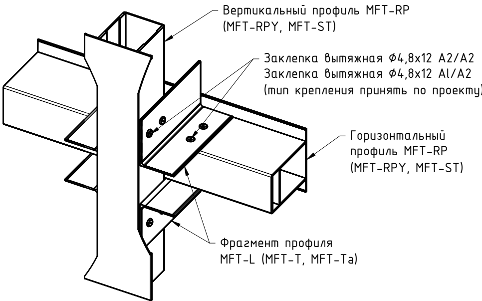
Узел №4 (увеличено)
