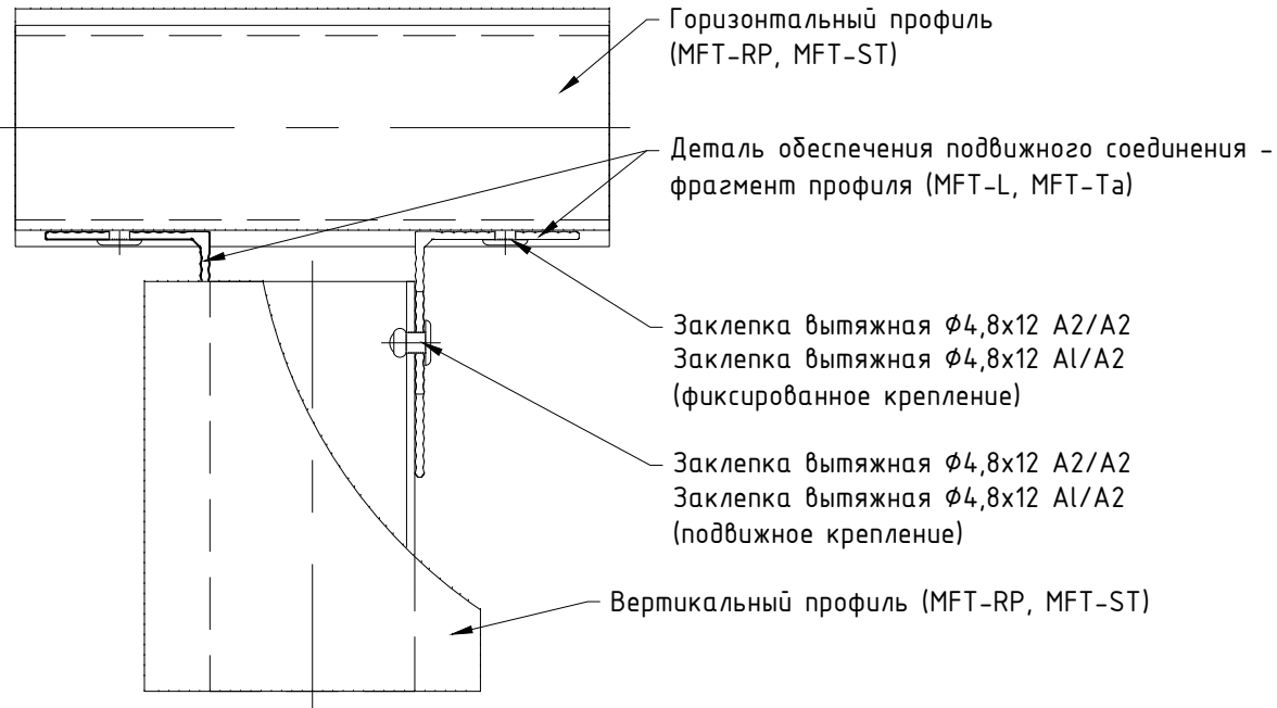
Узел №2 (увеличено)
