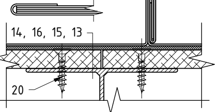
Сечение Б-Б
