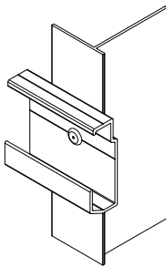
горизонтальные профили: MFT-HPE вертикальная направляющая: MFT-Ta
