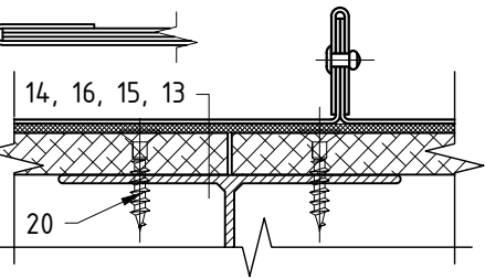
Сечение Б-Б
