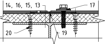
Сечение А-А (вар. 3)
