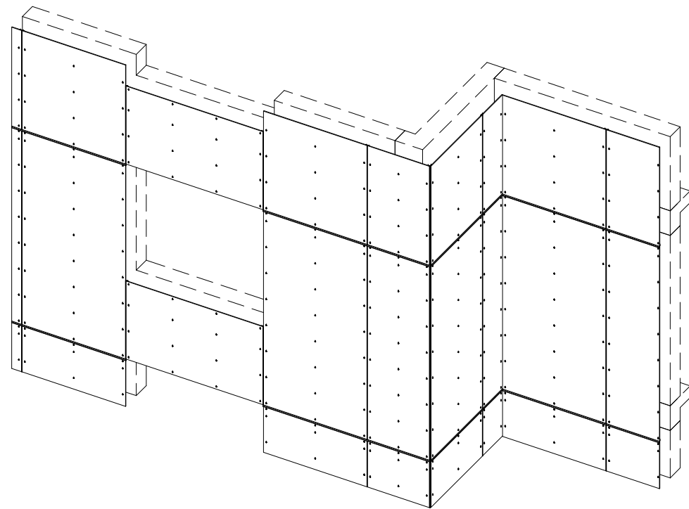
HPL-панель, скрытое крепление: горизонтальное расположение
