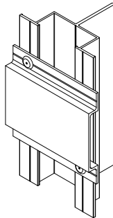
горизонтальные профили: MFT-HPE вертикальная направляющая: MFT-Y
