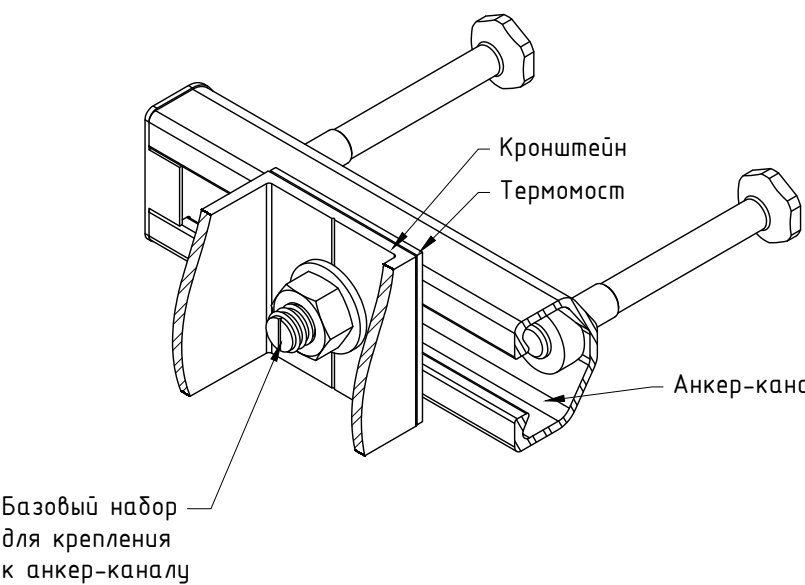
Пример крепления П-образных кронштейнов с одним отверстием в основании.
