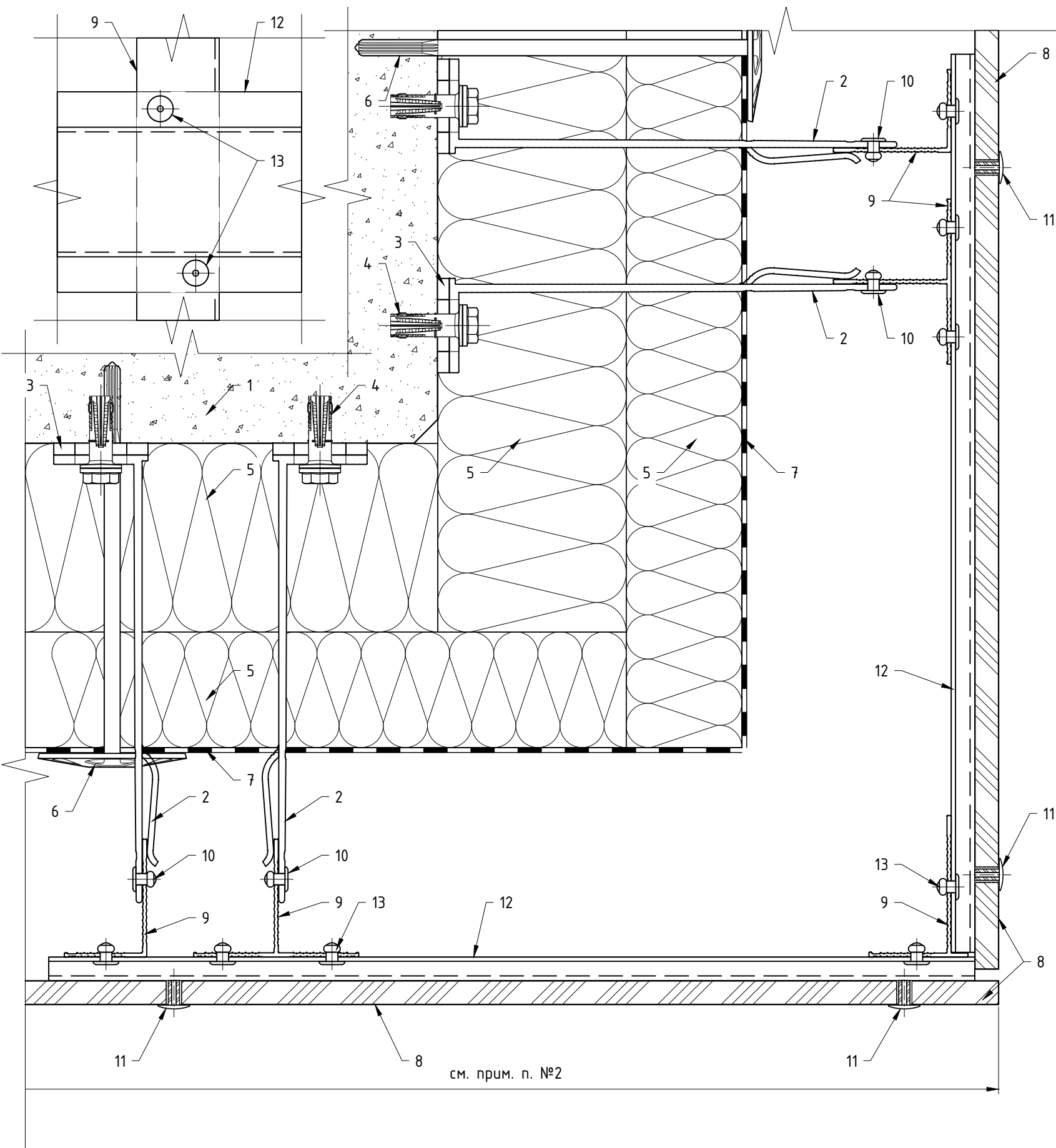
Выполнение наружного угла фасада: элементы "Light", вертикальная схема расположения элементов системы, видимое крепление на заклепки, вариант №4.
